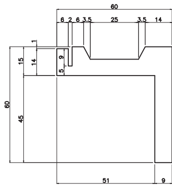
62 t 用D枠
