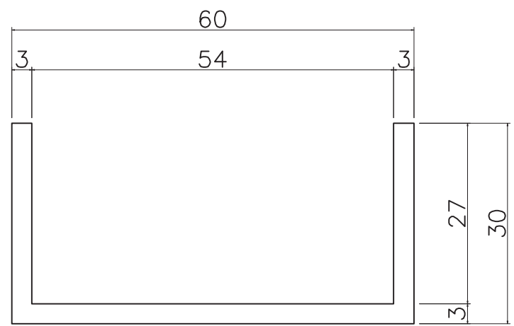
アルミチャンネル 定尺寸法 L = 3800
