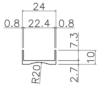
10×24×10 定尺寸法 L=6000
