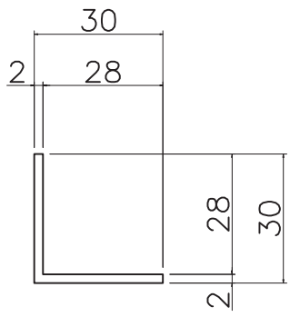
2.0t×30×30 定尺寸法 L=4000 (アルマイト処理)
