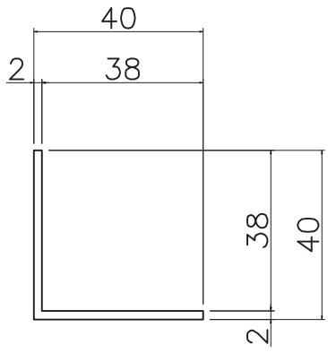
2.0t×40×40 定尺寸法 L=4000 (アルマイト処理)
