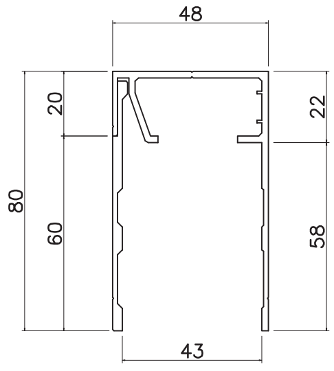
アルミ上部レール 42-TP80 (シルバー) 定尺寸法 L=2700
